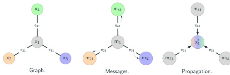
شکل (۳): محاسبه لایه‌های پنهان شبکه
