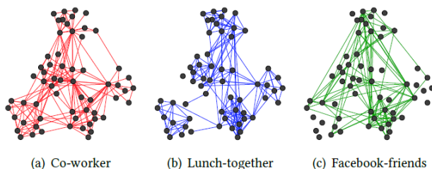
شکل ۲: نمونه‌ای از شبکه‌ی مولتی-پلکس
